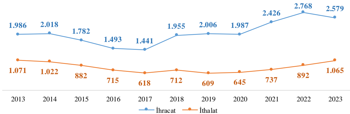
Grafik 57 - KOBİ’lerde 23- Diğer Metalik Olmayan Mineral Ürünler Ürün Grubu İhracat ve İthalatı (Milyon ABD $)
